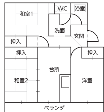
横落住宅間取図
