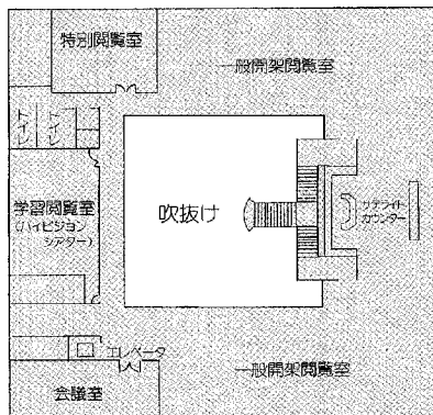
2階平面図
