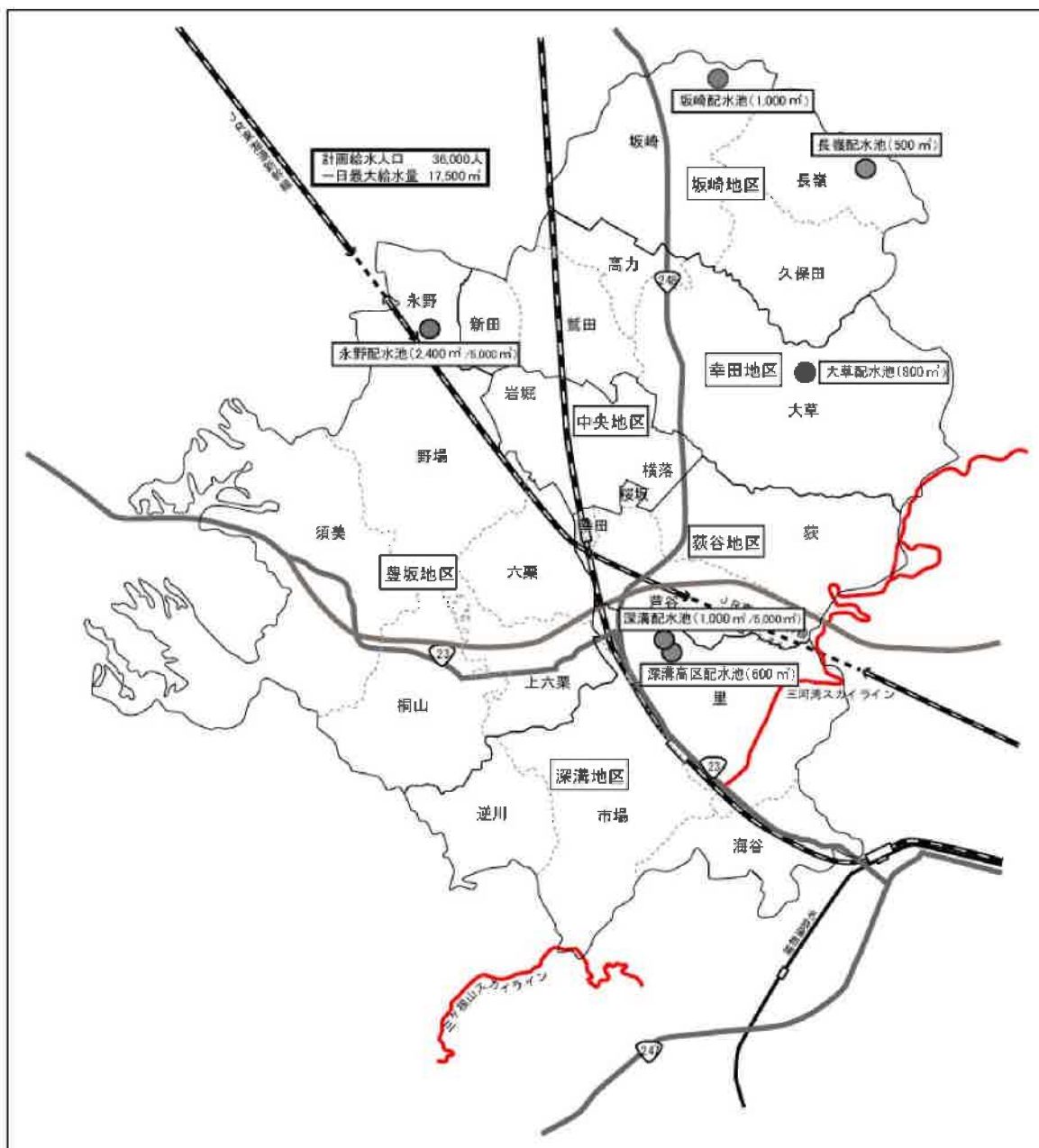
図4-6 配水池
