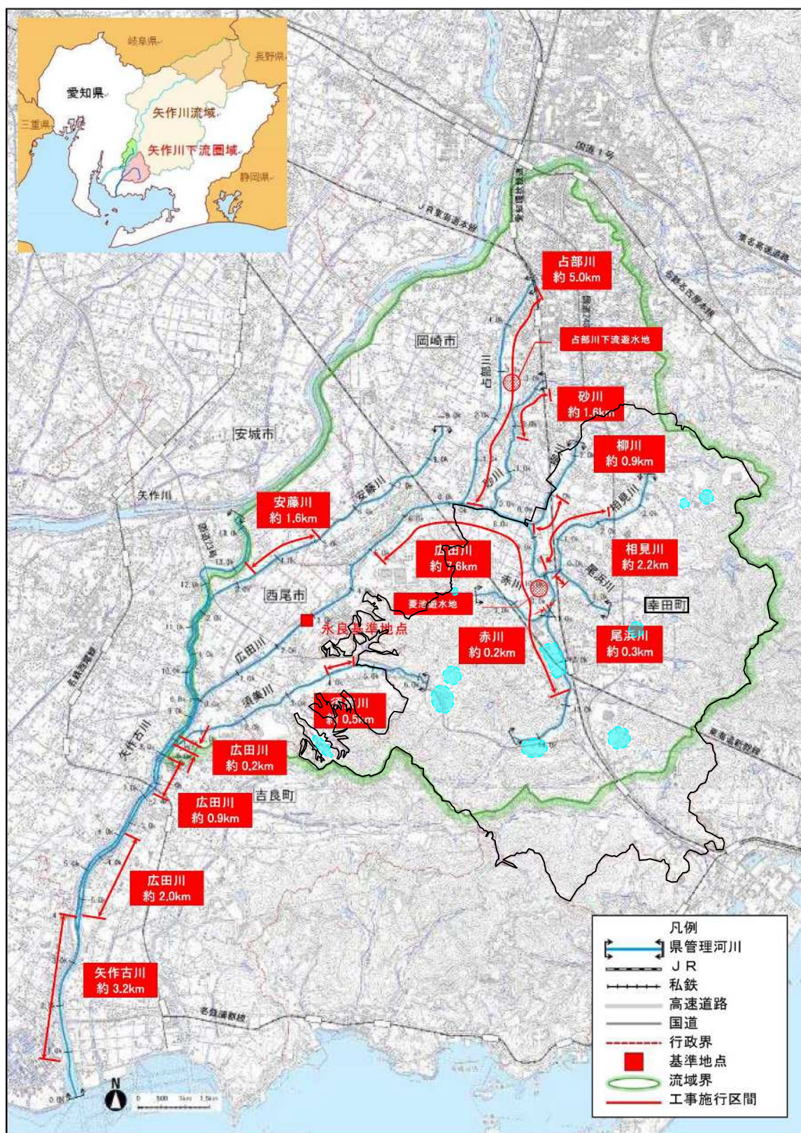
■矢作川下流圏域河川整備計画図（平成 28 年 6 月 3 日一部変更）
