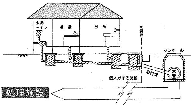
農業集落排水処理施設のしくみ
