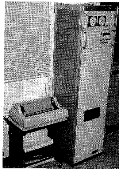
▲総合気象観測盤(観測器のメイン)
