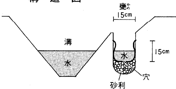
構造図
