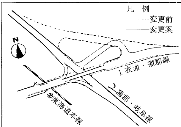
3, 4は附加車線
