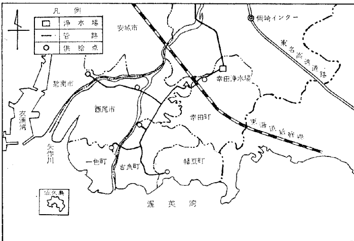
西三河水道用水供給事業概要図(幸田浄水場関係分)
